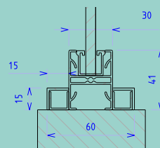
Coupe verticale Par défaut
