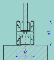
Coupe verticale Option gratuite
