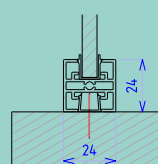
Coupe verticale Par défaut standard Option gratuite sur-mesure
